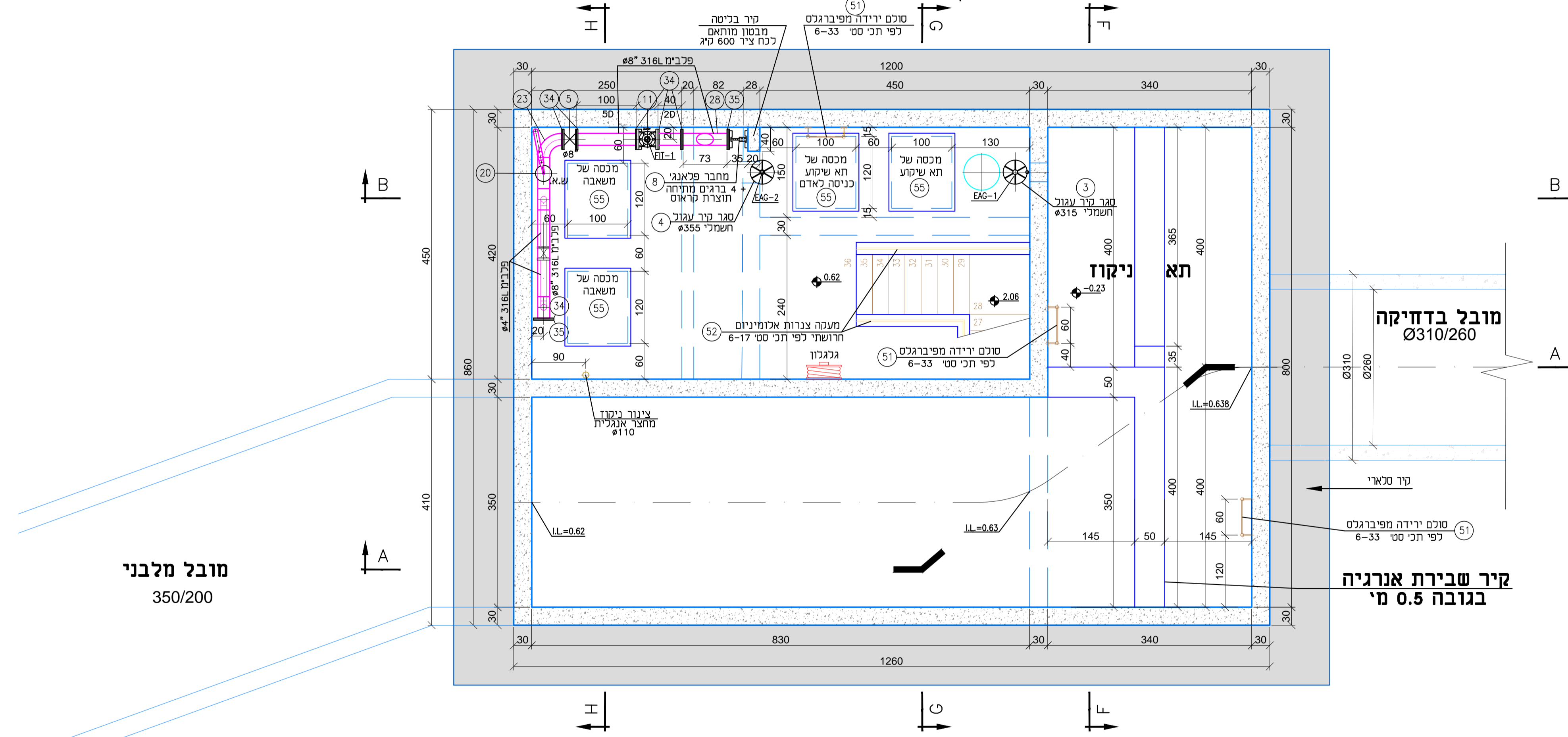
תכנית במפלסים -2.26, -1.68, -0.23 חתך C-C
