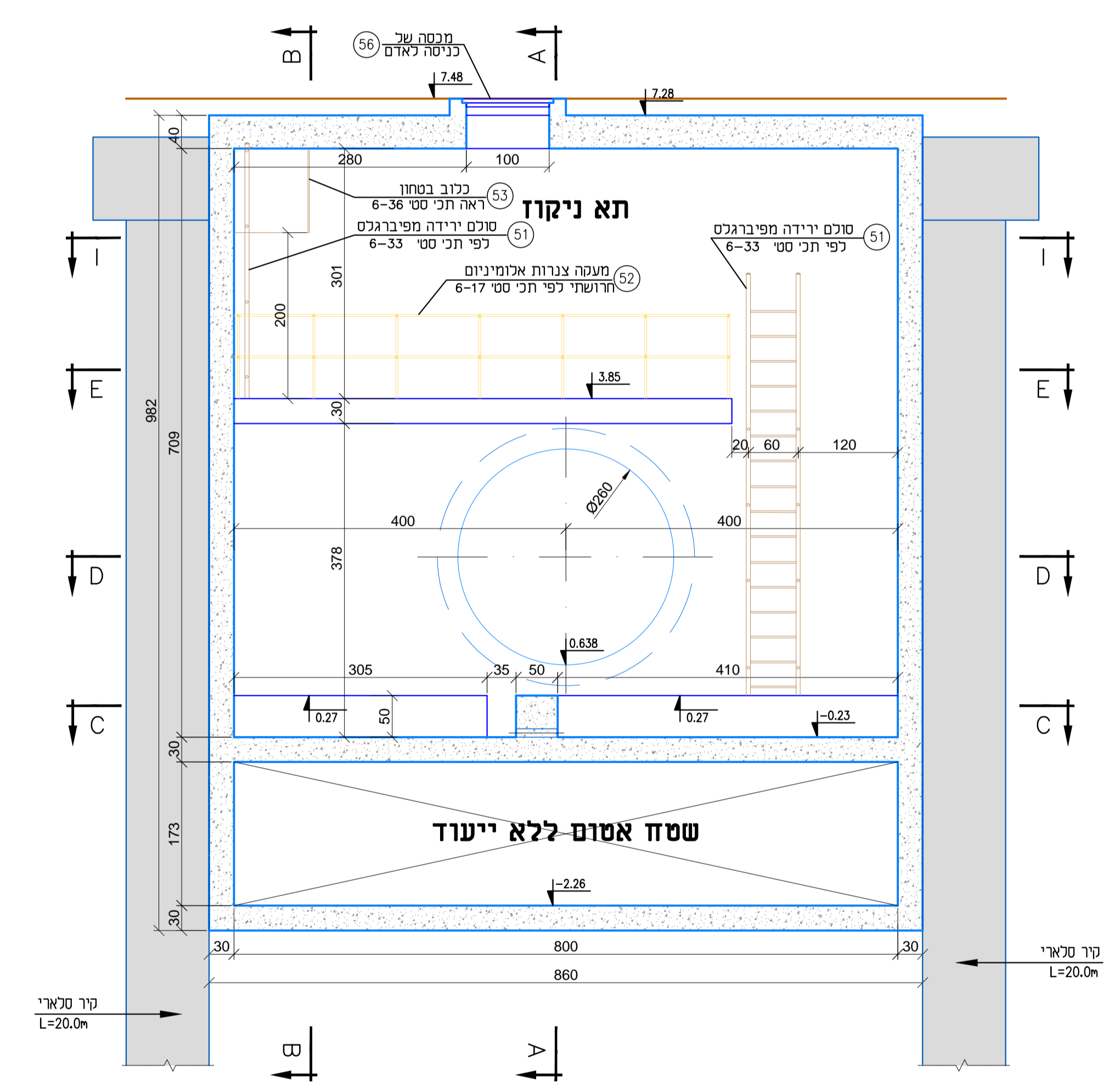
חתך F-F מידות בט"מ
