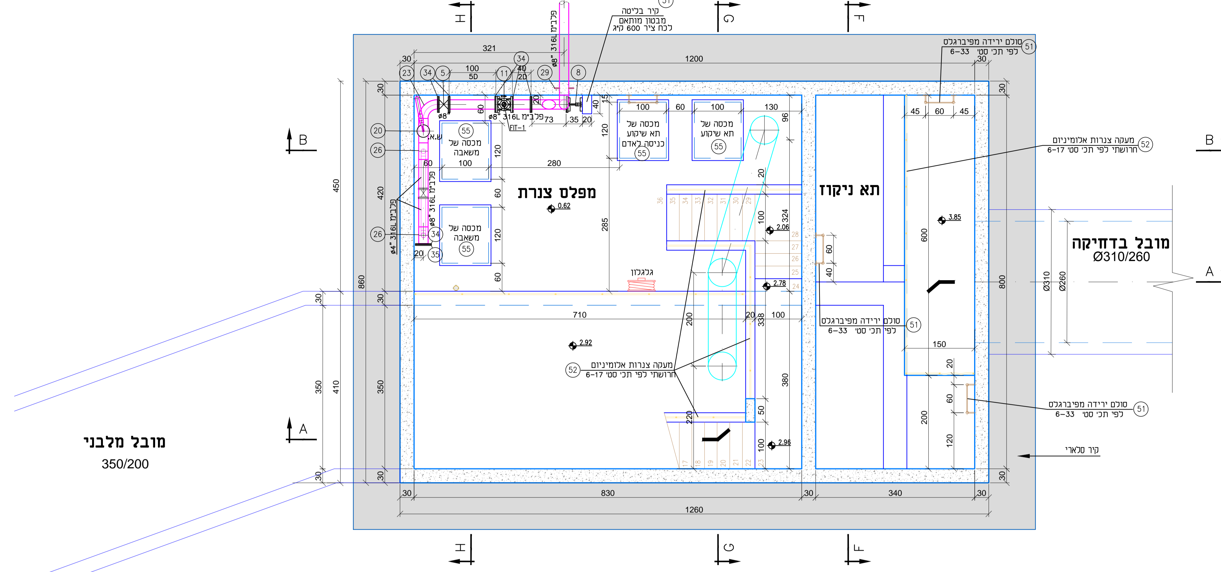
תכנית במפלס 0.62 חתך D-D
