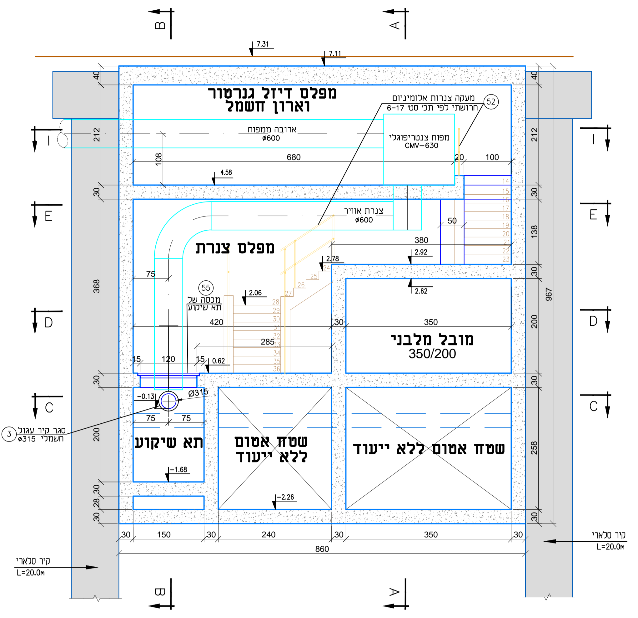
חתך G-G מידות בט"מ
